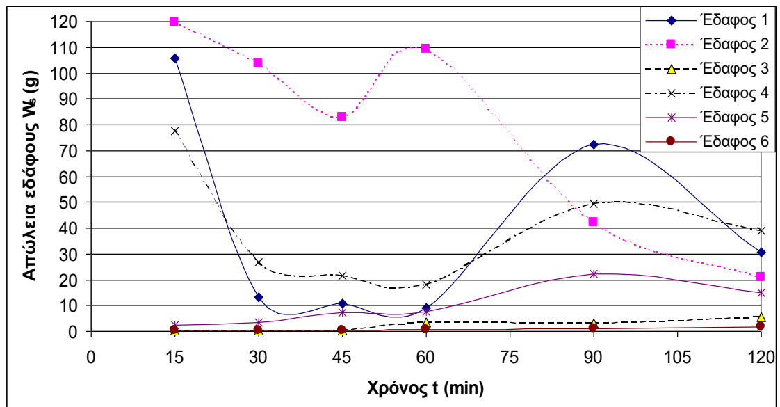
Σχήμα 1.1: Μεταβολή της απώλειας λόγω διάβρωσης έξι εδαφών με το χρόνο
